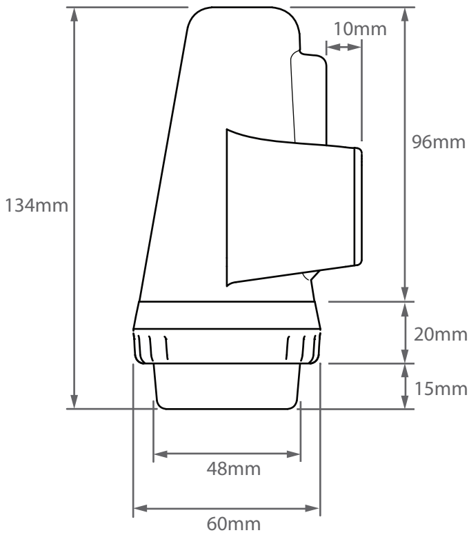
LS1-R Dimensions
